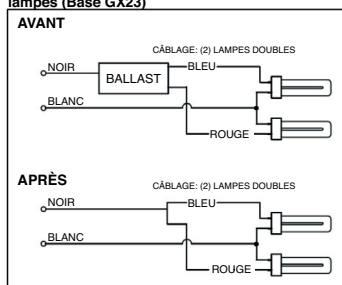
Figure 2. Modernisation avec deux lampes (Base GX23)
